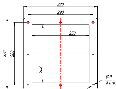
Выходной фланец
