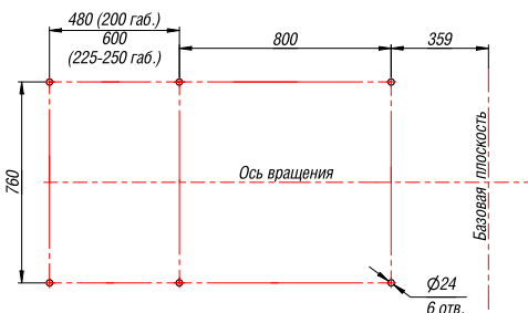
Схема расположения отверстий для крепления вентилятора
