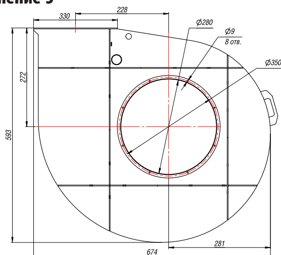
Выходной фланец
